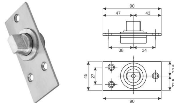
DM-502D : Bottom Door Patch Insert
