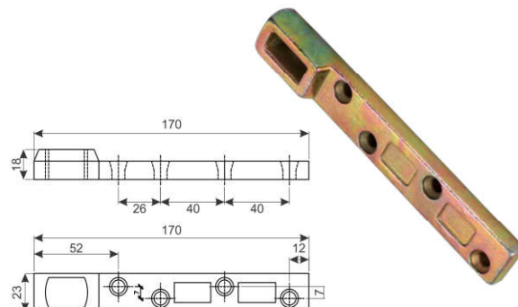
DM-502M : Bottom Door Patch Insert
